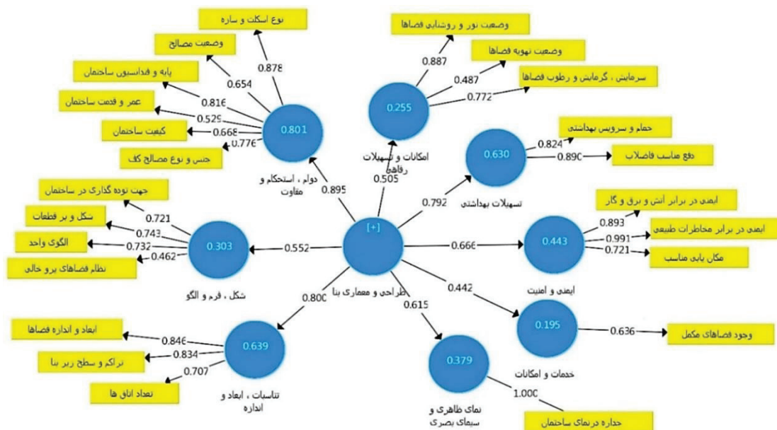
تصویر ۲- مدل‌سازی مسیری PLS
