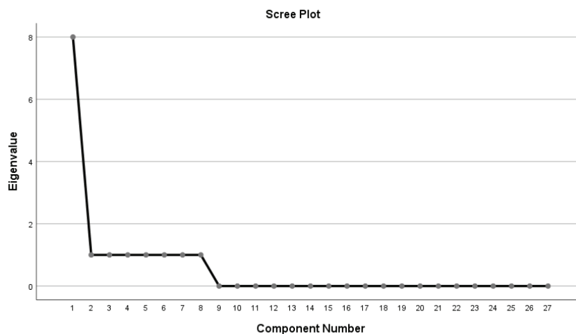
تصویر ۳- نمودار اسکری پلات
