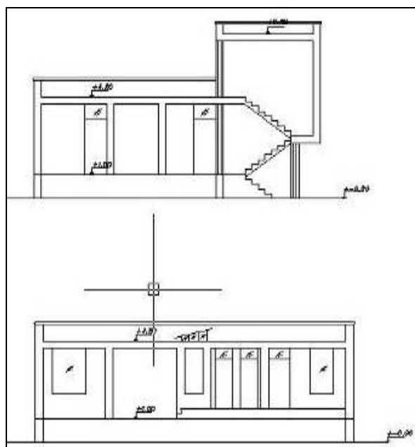
تصویر ۹- پلان مربوط به مسکن روستایی با طرح منزل اعیانی و دوطبقه در روستای چمگل (۵۷-۱۳۴۲)
