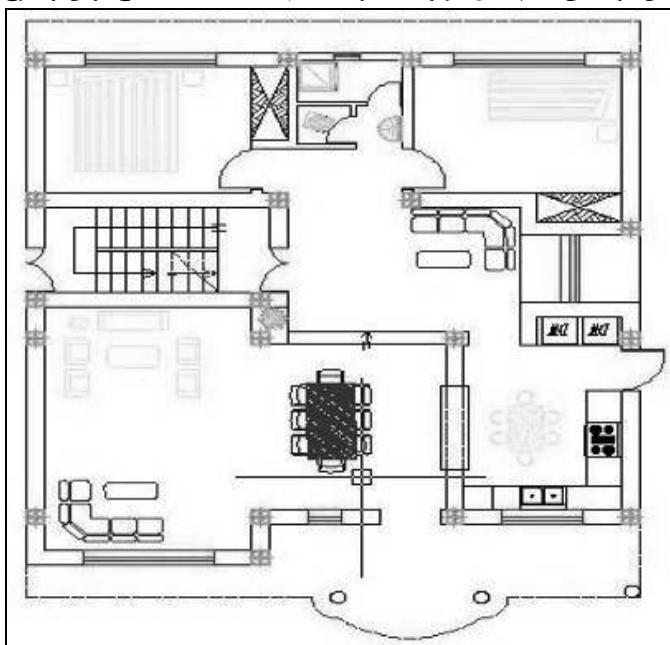
تصویر ۱۵- پلان و چیدمان درونی مسکن روستایی در دوره ششم بر اساس الگوی مدرن (۹۱-۱۳۸۰)
