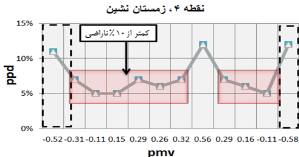
تصویر ۶- نمودار PPD محاسبه شده نقاط در ساعات مختلف
