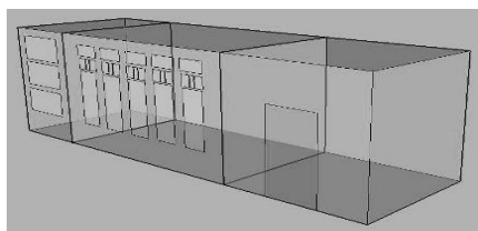
تصویر ۳- شبیه‌سازی و بندی Zone بندی (اتاق زمستان نشین خانه تولایی)
