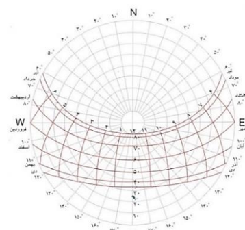
تصویر ۳، موقعیت و زوایای تابش خورشید طبق عرض جغرافیایی ۳۵ درجه شمالی؛ منبع کسمایی
