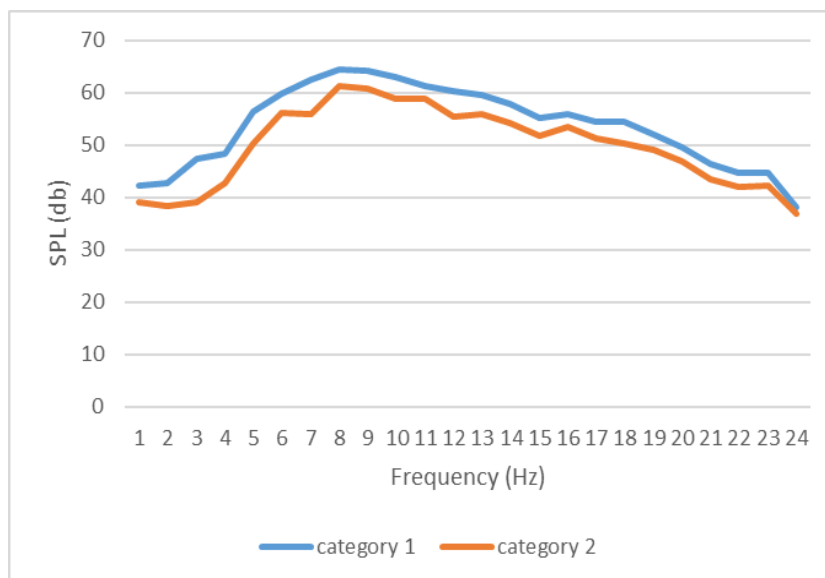
تصویر ۷- مقایسه میانگین تراز فشار صوتی حاکم در اتاق های خواب در دسته بندی ۱ (مکان یابی عرصه خدماتی در کنار اتاق های خواب) و دسته بندی ۲ (مکان یابی عرصه خدماتی در کنار نشیمن و پذیرایی و به دور از عرصه استراحتی مسکن)
