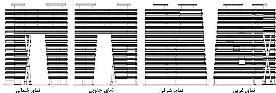
تصویر ۱۱- نمای برج‌های مسکونی پزشکان آبخار را در چهار جبهه مختلف
