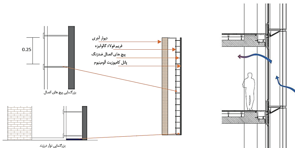
تصویر ۶- جزئیات اجرایی پوسته دوم و نحوه اتصال به پوسته اصلی
