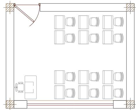
تصویر ۲۱ و ۲۲- میزان سایه اندازی طرح آزمایشی برای کلاس درس با بازو جنوبی
