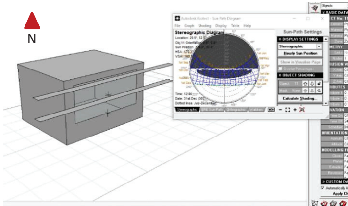
تصویر ۲۱ و ۲۲- میزان سایه اندازی طرح آزمایشی برای کلاس درس با بازو جنوبی
