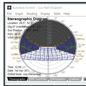
تصویر ۲۳- شرایط فعلی سایه اندازی سایه بان های کلاس های درس با بازو جنوبی
