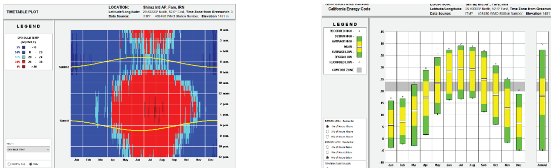
تصوير ۱- حداقل و حداكثر دما در ماه‌هاى سال در شيراز در نرم‌افزار اكوكتك تصوير ۲- دما در ماه‌هاى سال از طلوع تا غروب در نرم‌افزار اكوكتك
