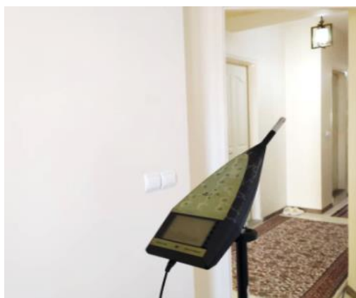
تصویر ۲- نمونه‌ای از دستگاه آنالیز صوتی ۲۲۶۰ در حین انجام آزمایشات صوتی در داخلی یکی از واحدهای مسکونی
