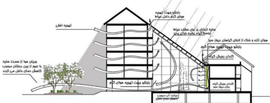
کاربرد تابستانی حیاط مرکزی
