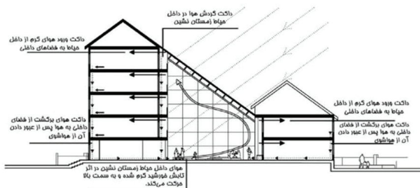
کاربرد زمستانی حیاط مرکزی و نحوه گردش هوا در داخل آن
