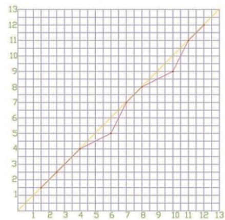
تصویر ۶- مختصات ابعاد بهینه نورگیر در اعتدال بهاری
